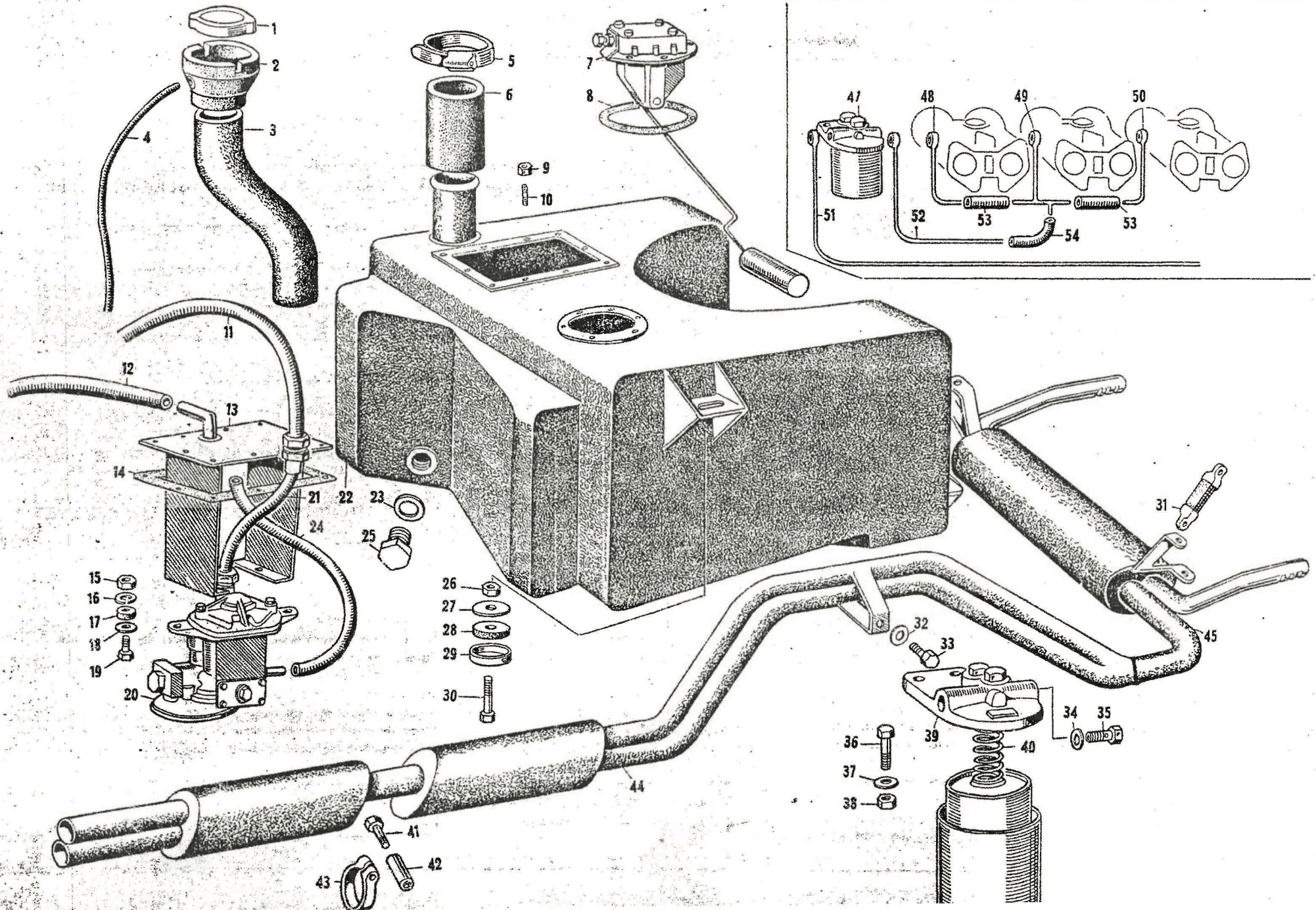
Tavola 32 - Tubo di scarico e serbatoio benzina
