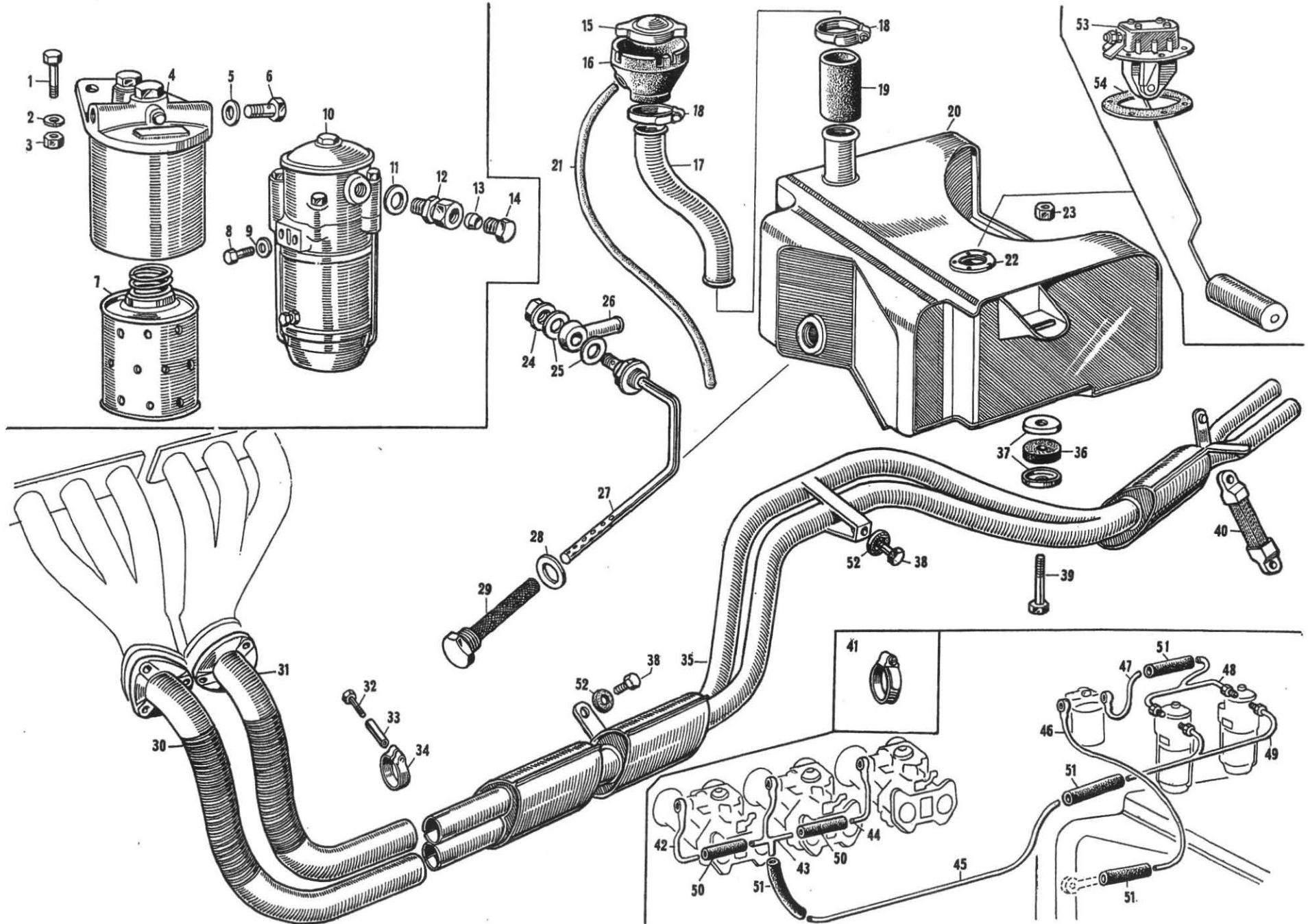
Tavola 11 - Tubo di scarico e serbatoio benzina
