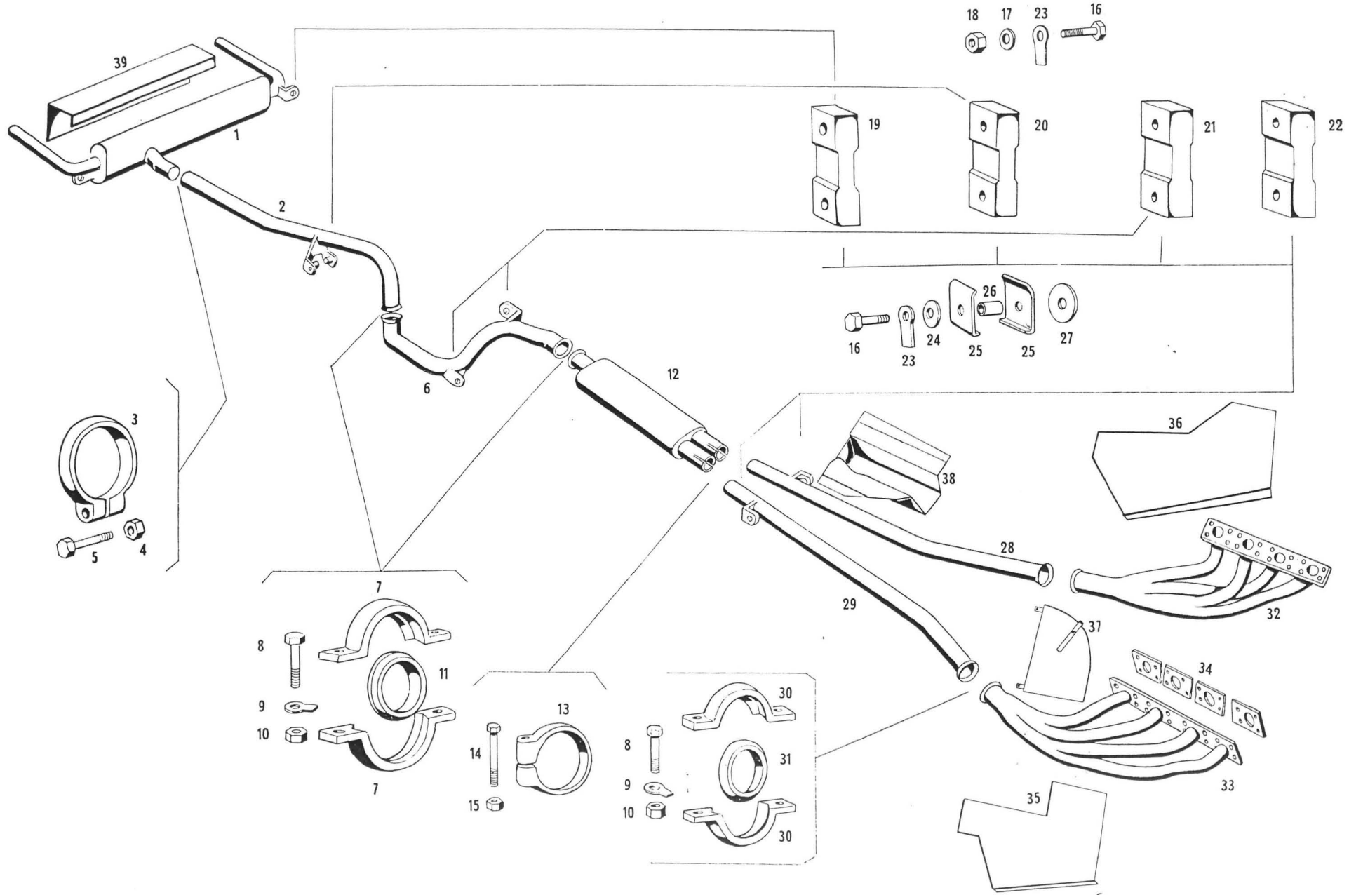
Tavola 28 - Tubi di scarico Table 28 - Exhaust pipes
