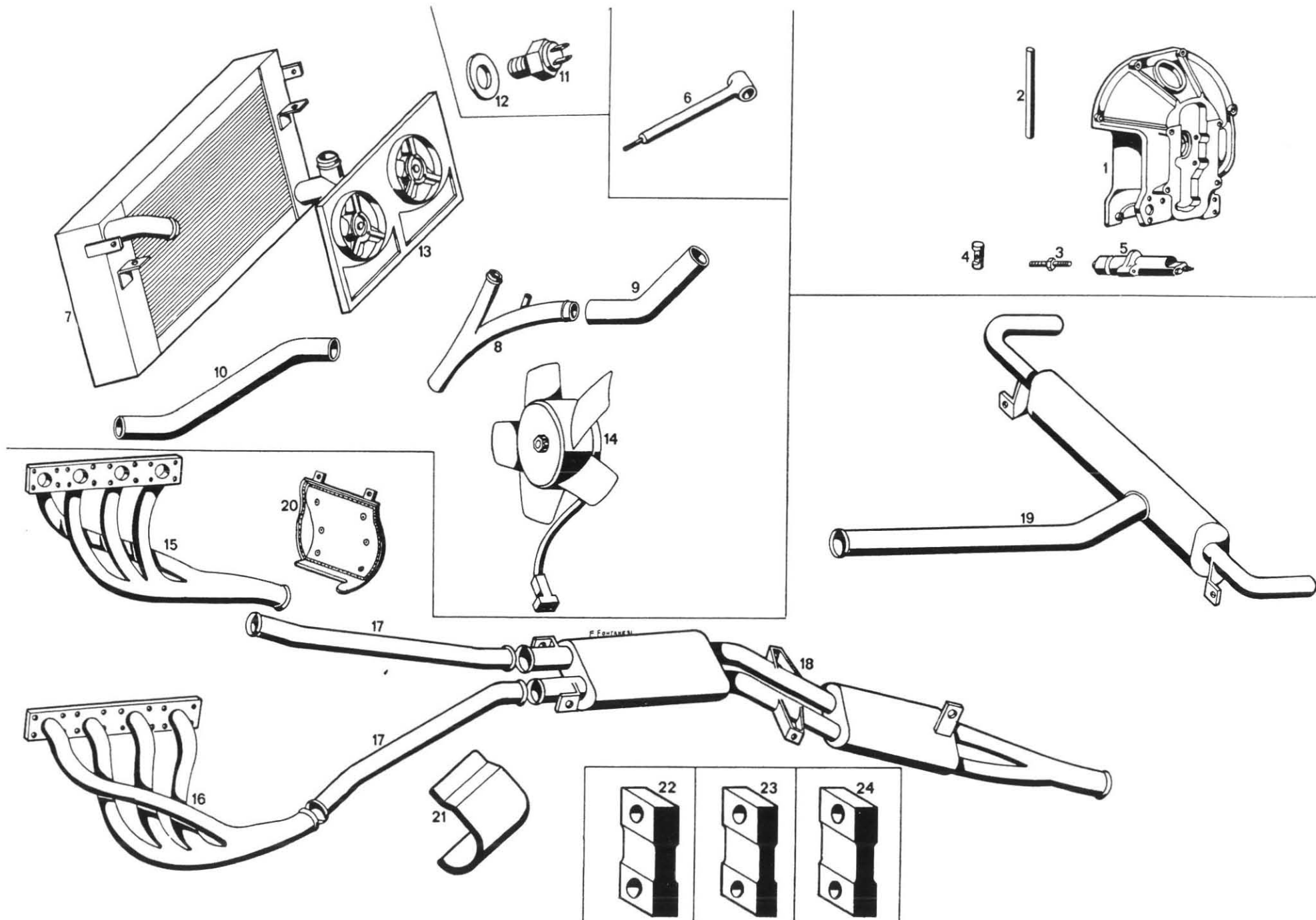
TAVOLA 3 - RAFFREDDAMENTO SCARICHI E FRIZIONE TABLE 3 - ENGINE COOLING EXHAUST PIPES AND CLUTCH
