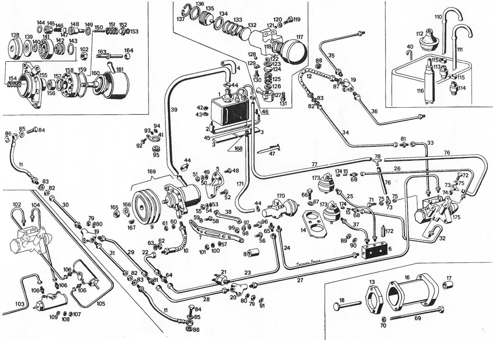
TAVOLA 9 - CIRCUITO FRENANTE TABLE 9 - BRAKE CONTROL
