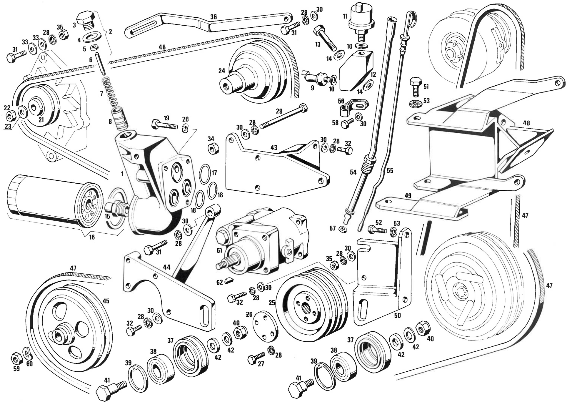
Tavola 6 - Cinghie e pulegge Table 6 - Belts and pulley
