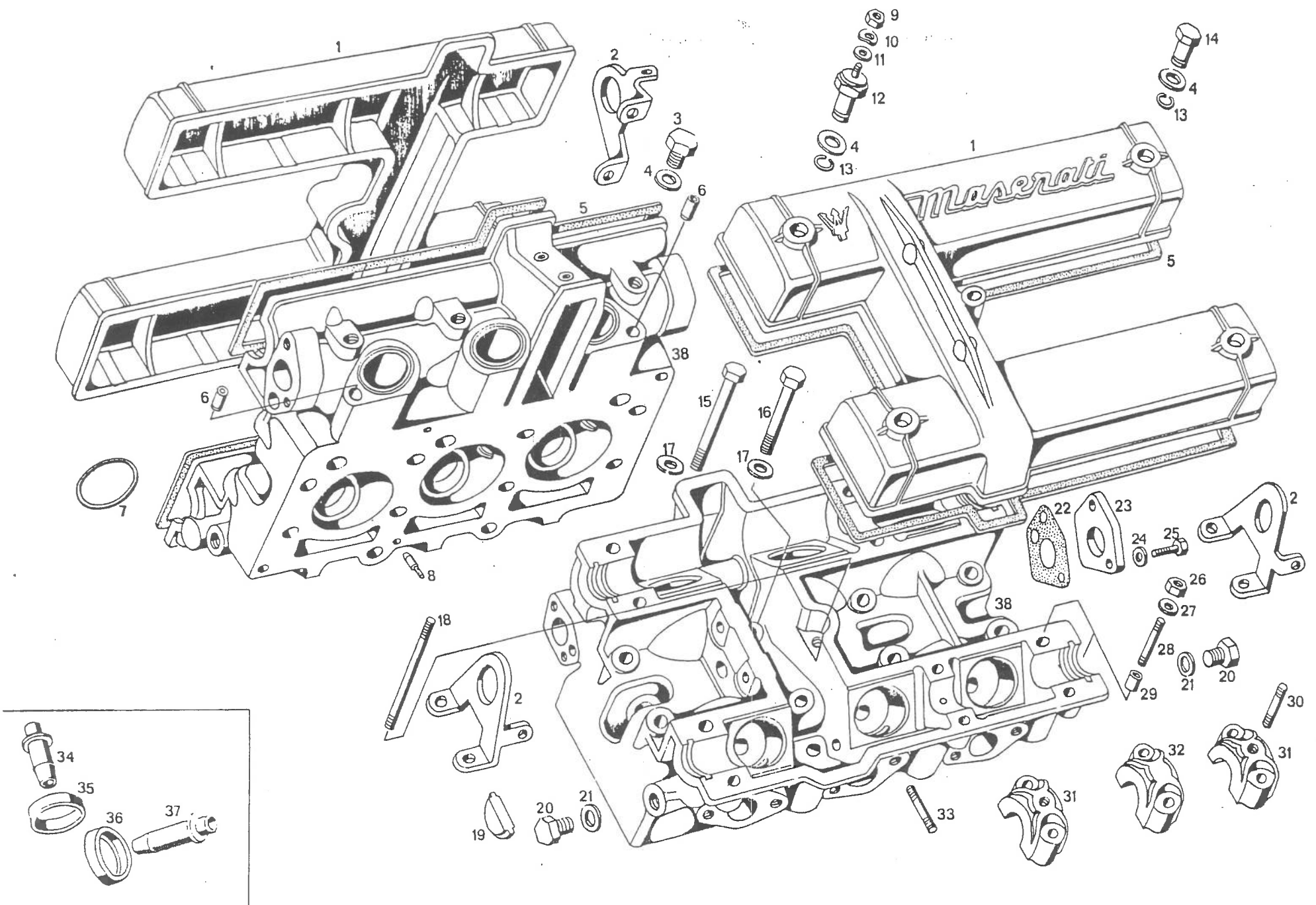
Tavola 1 - Teste cilindri Tafel 1 - Zylinder Köpfe
