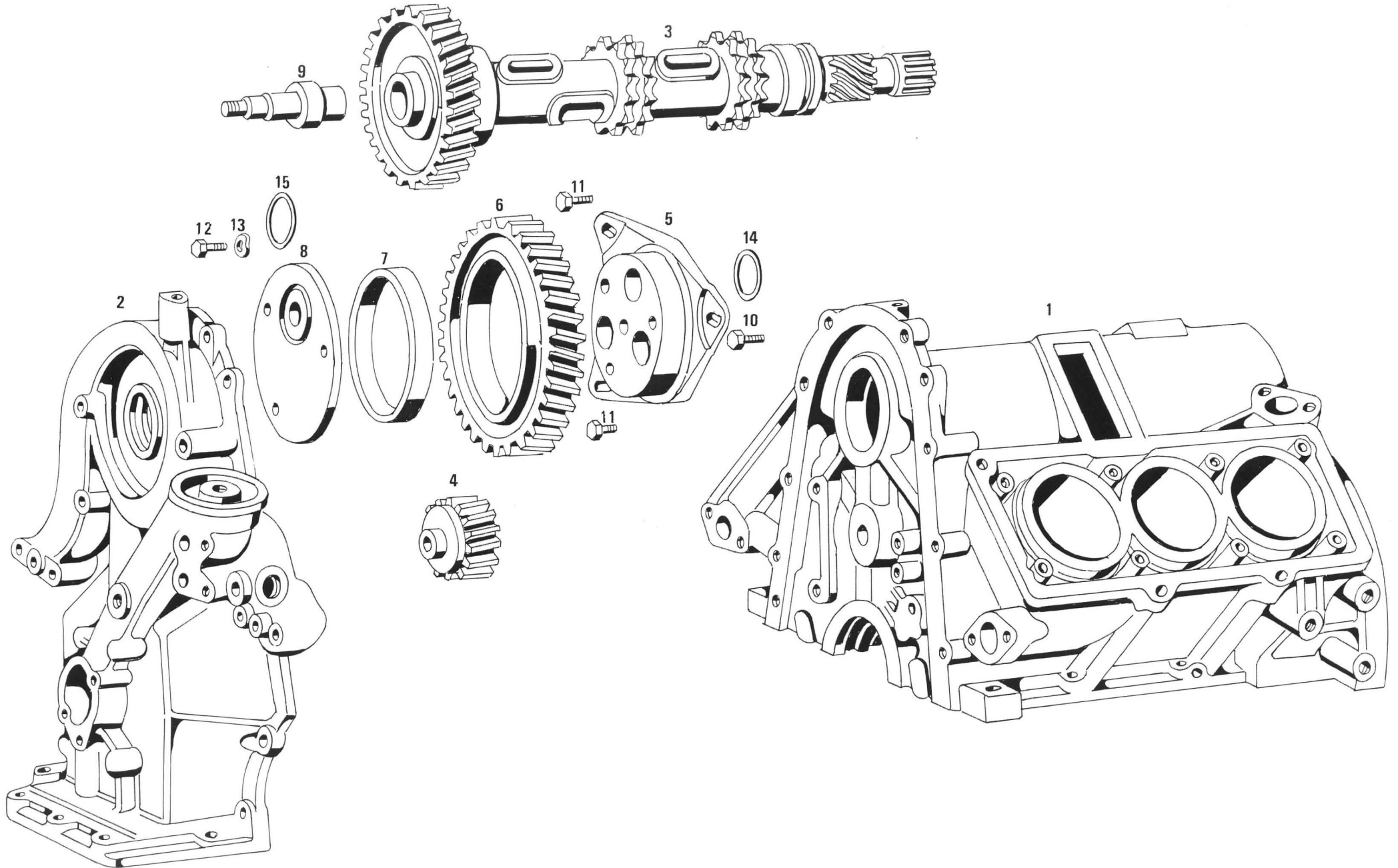
Tavola 2 - Distribuzione ad ingranaggi Table 2 - Distribution gear
