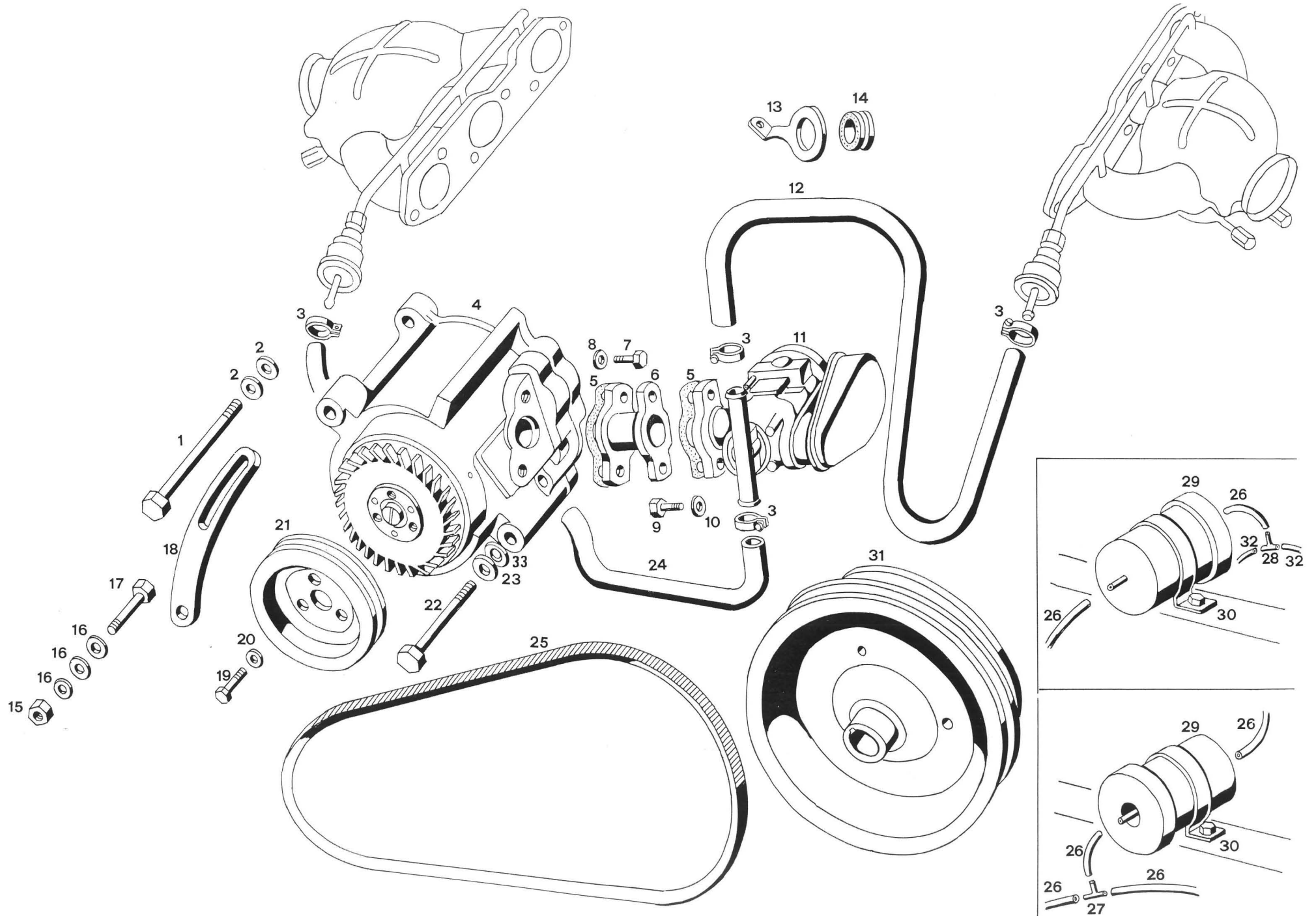
Tavola 5 - Pompa aria Table 5 - Air pump
