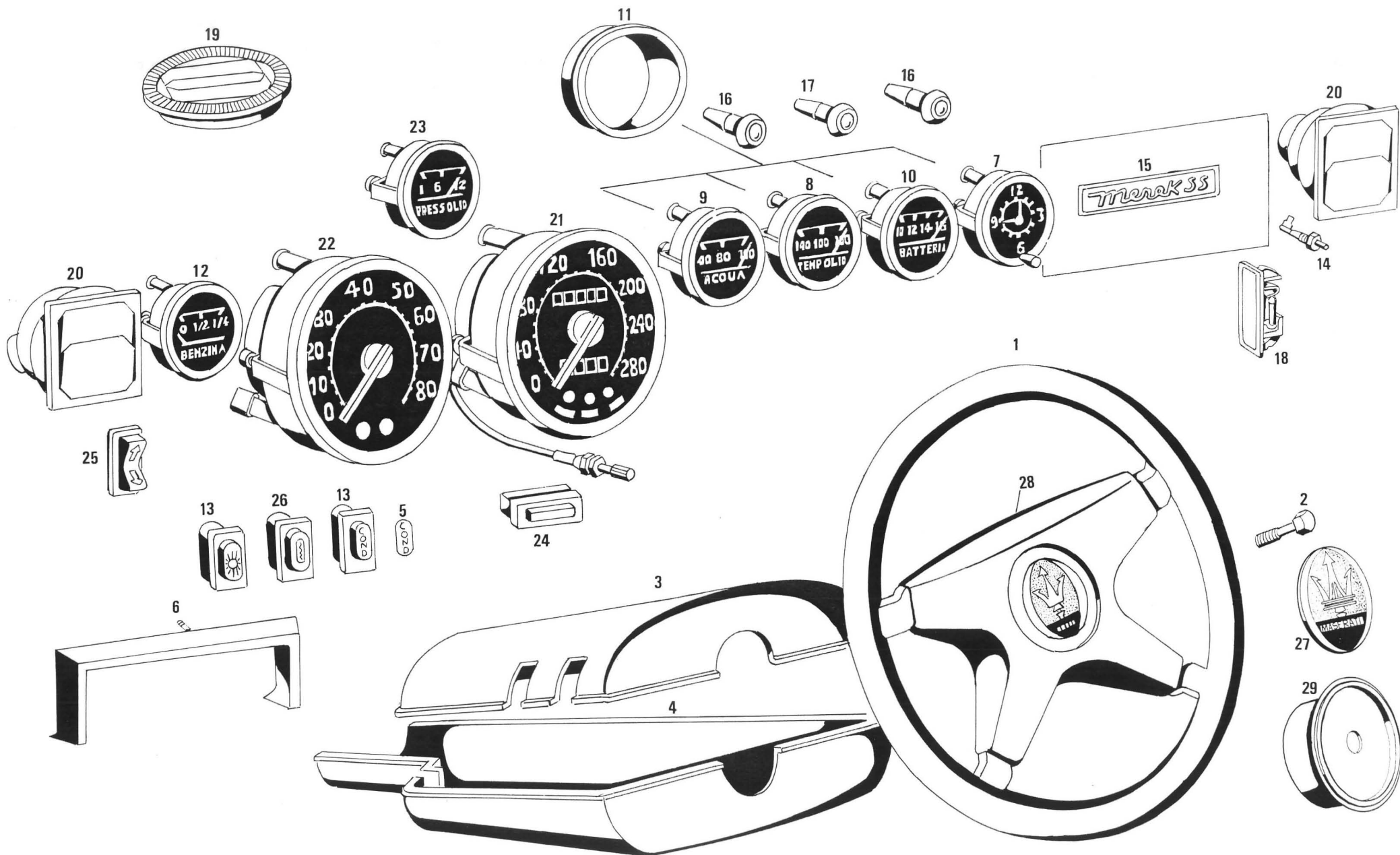
Tavola 17 - Strumenti cruscotto Table 17 - Dashboard Instruments
