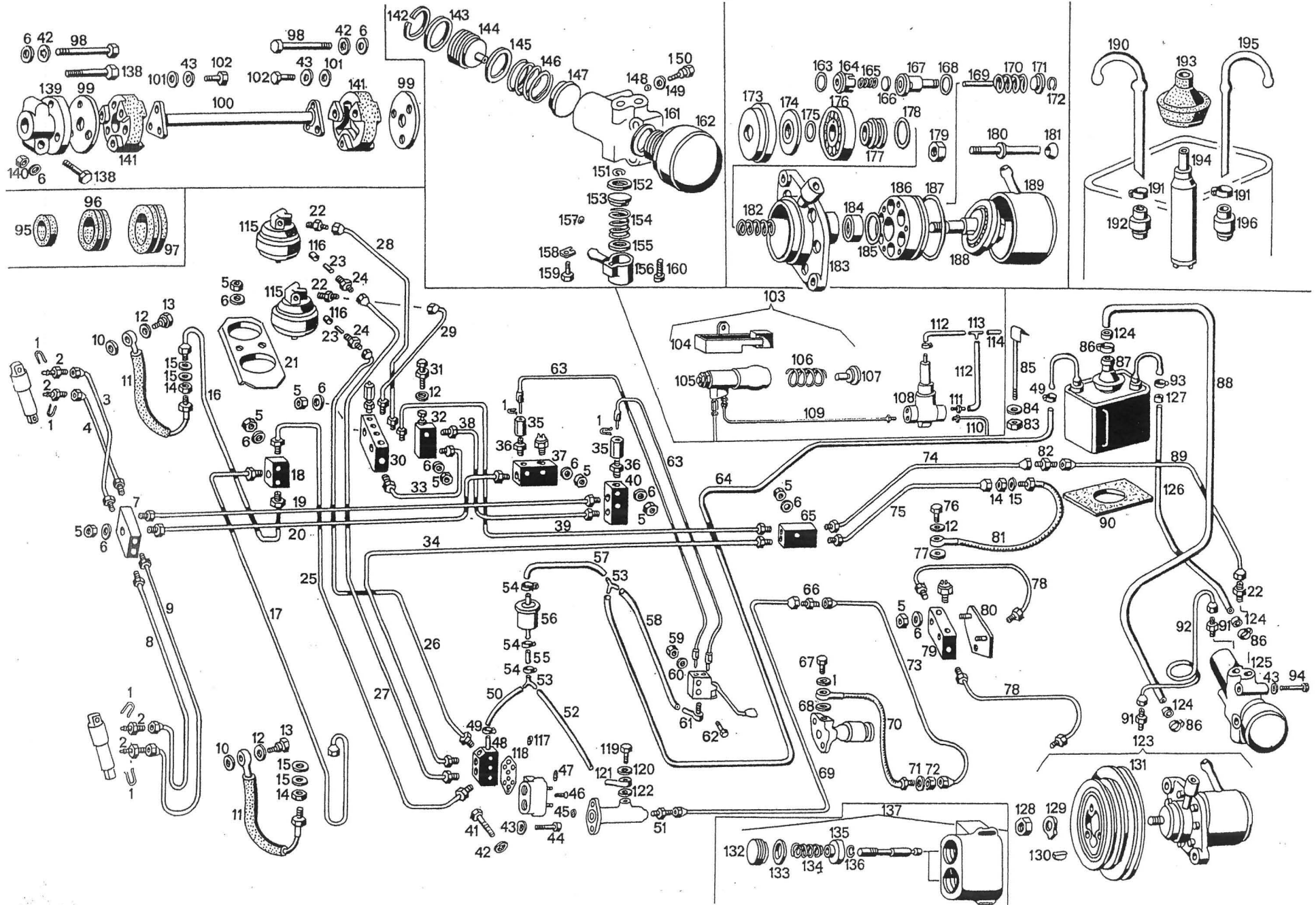
Tavola 23 - Circuito idraulico Table 23 - Braking system
