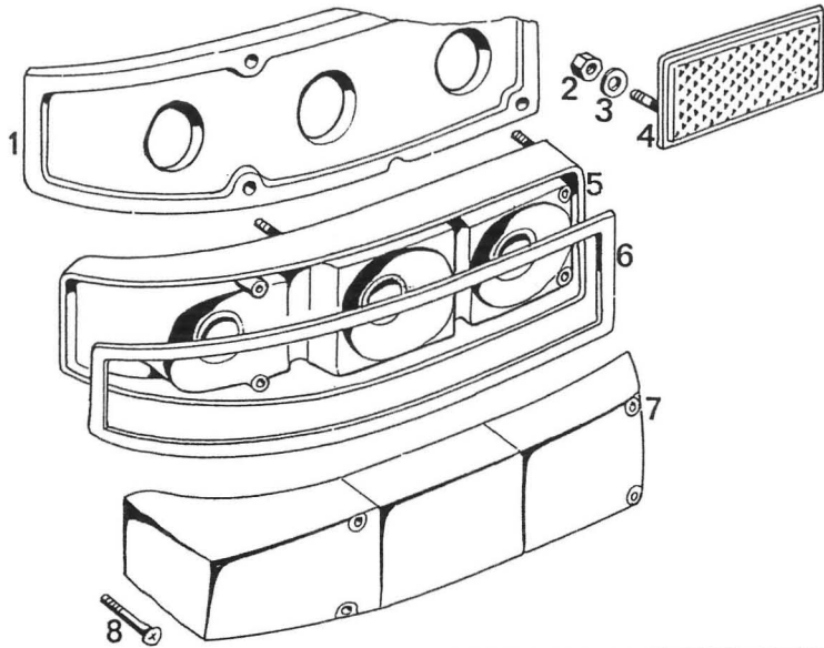
TAVOLA 3-EQUIPAGGIAMENTO ELETTRICO TABLE 3-ELECTRIC EQUIPMENT
